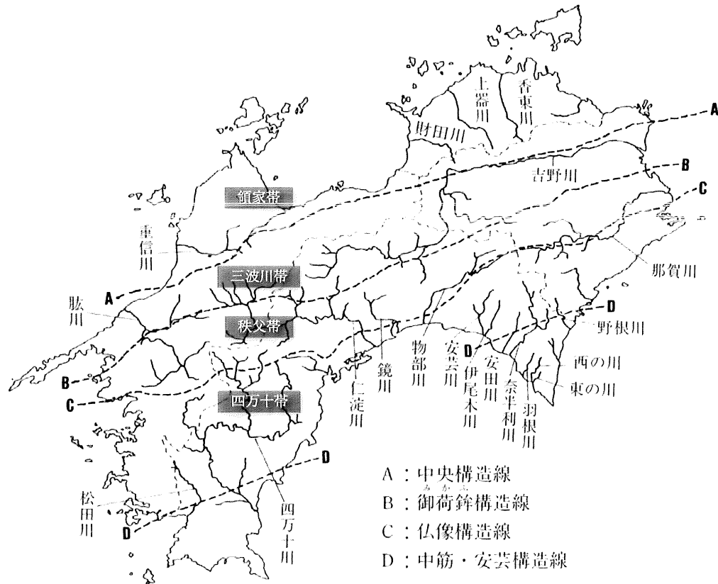
図 1-4 四国の地質構造線と河川
